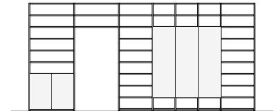
LIVING_427 Dimensione_size L 615,4 H 294,6 P 34
