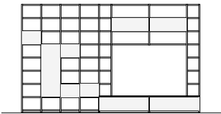
LIVING_429 Dimensione_size L 433,6 H 262,6 P 34/46,8
