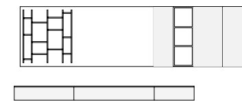
LIVING_432 Dimensione_size L 360 H 190 P 16,8/34/46,8
