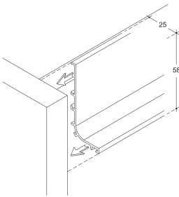
Battuta fianco terminale anta base / Single horizontal c-shaped groove leaned against end side panel / Горизонтальная одиночная изогнутая Gola до боковины.
