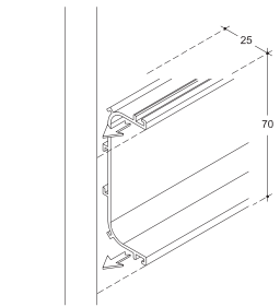
Battuta fianco terminale cestoni base / Double horizontal c-shaped groove leaned against end side panel / Горизонтальная двойная изогнутая Gola до боковины.
