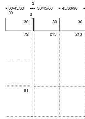
SOPRAPENSILE - 1 ANTA / OVERHANGING WALL UNIT - 1 DOOR / АНТРЕСОЛЬ - 1 ДВЕРЬ SOPRACOLONNA CON ANTE / OVERHANGING TALL UNIT WITH DOORS / СОПРАКОЛОННА С ДВЕРЯМИ
