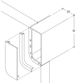
Passante fianco terminale anta base / Single horizontal flat groove placed on end side panel / Горизонтальная одиночная плоская Gola на боковине.
