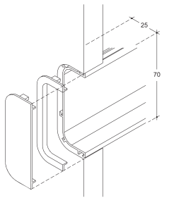
Passante fianco terminale cestoni base / Double horizontal c-shaped groove placed on end side panel / Горизонтальная двойная изогнутая Gola на боковине.
