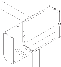
Passante fianco terminale anta base / Single horizontal c-shaped groove placed on end side panel / Горизонтальная одиночная изогнутая Gola на боковине.
