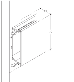
Battuta fianco terminale cestoni base / Double horizontal flat groove leaned against end side panel / Горизонтальная двойная плоская Gola до боковины.
