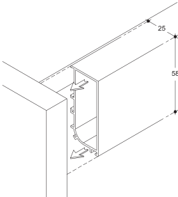
Battuta fianco terminale anta base / Single horizontal flat groove leaned against end side panel / Горизонтальная одиночная плоская Gola до боковины.
