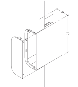
Passante fianco terminale cestoni base / Double horizontal flat groove placed on end side panel / Горизонтальная двойная плоская Gola на боковине.
