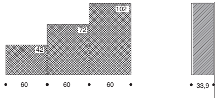
PENSILE - ANTA VETRO SERIGRAFATO / WALL UNIT - SERIGRAPHY GLASS DOOR / НАВЕСНЫЙ ШКАФ - ДВЕРЬ СО СЕРИГРАФИРОВАННЫМ СТЕКЛОМ
